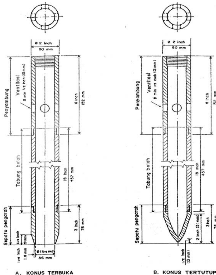
Gambar 1 Alat pengambilan contoh tabung belah
