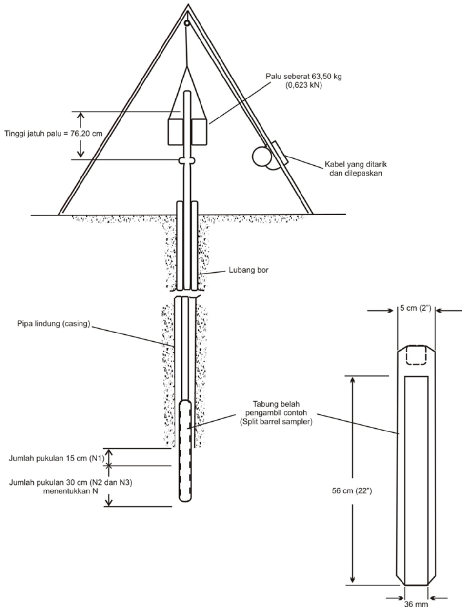
Gambar 2 Penetrasi dengan SPT
