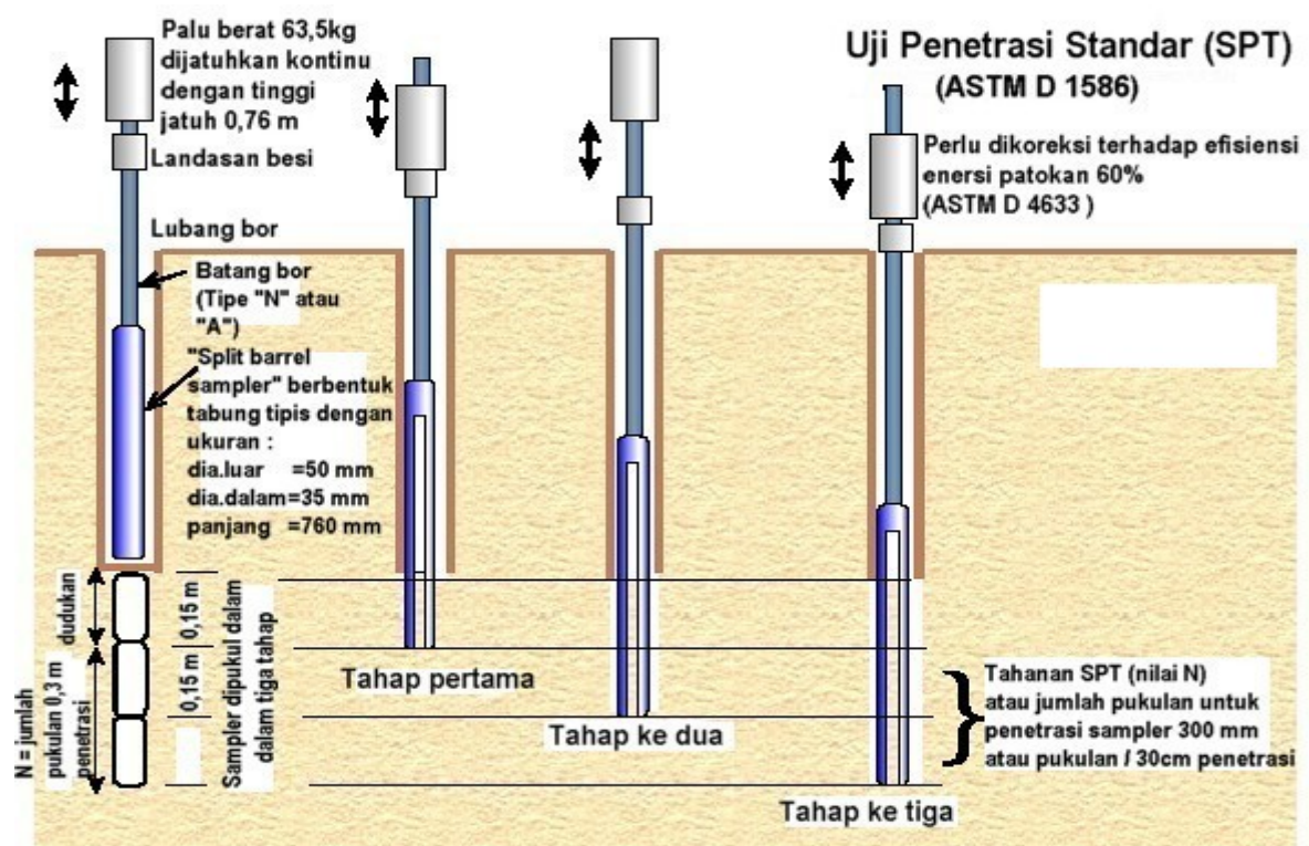
Gambar 3 Skema urutan uji penetrasi standar (SPT)
